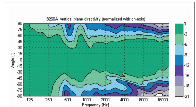
Abbildung 25: Darstellung der vertikalen Richtwirkung eines 8260A
