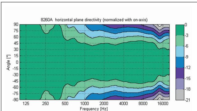
Abbildung 24: Darstellung der horizontalen Richtwirkung eines 8260A
