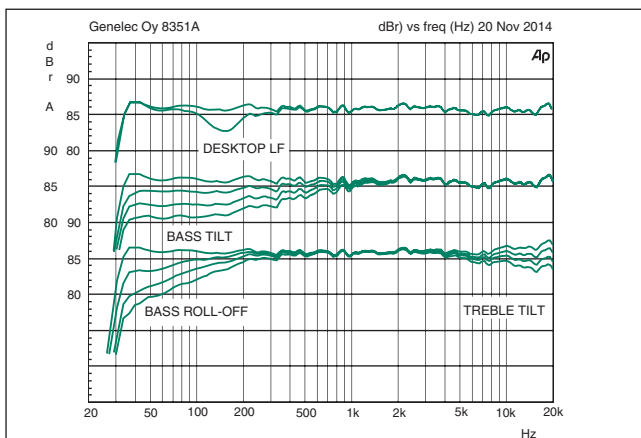
Abbildung 14: Die Kurven zeigen den Effekt der Schalter "Bass Tilt", "Treble Tilt", "Desktop Low Frequency" und "Bass Roll-Off" auf den Frequenzgang eines 8351A im Freifeld
